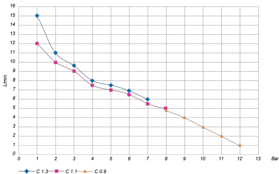
Krzywa wydajności
