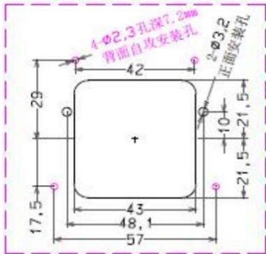
安装开孔图
