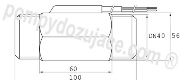
Rysunek techniczny
